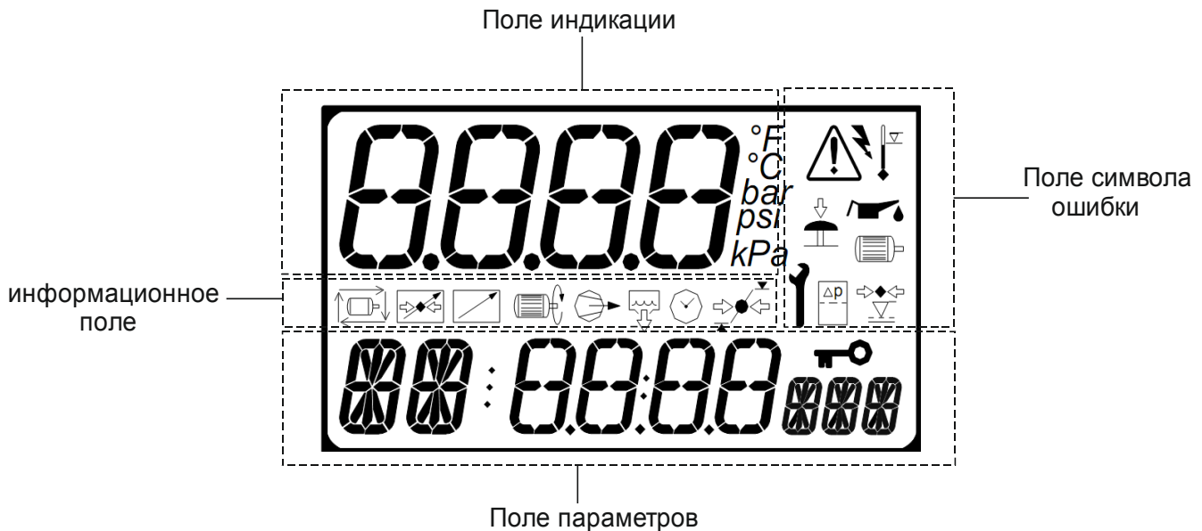
Рис. 1. Дисплей контроллера
